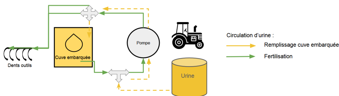
Figure 27 Schéma des flux d'urine dans le Pipiculteur
