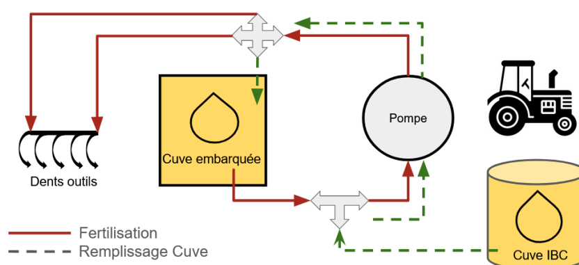
Figure 14 Schéma des flux de lisain dans le Pipiculteur
