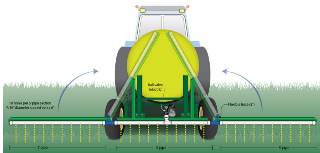
Figure 6 : Épandeur à urine stabilisée auto-construit par le Rich Earth Institute (Atlee 2019) à utiliser en grandes cultures et prairies. Source : Rich Earth Institute
