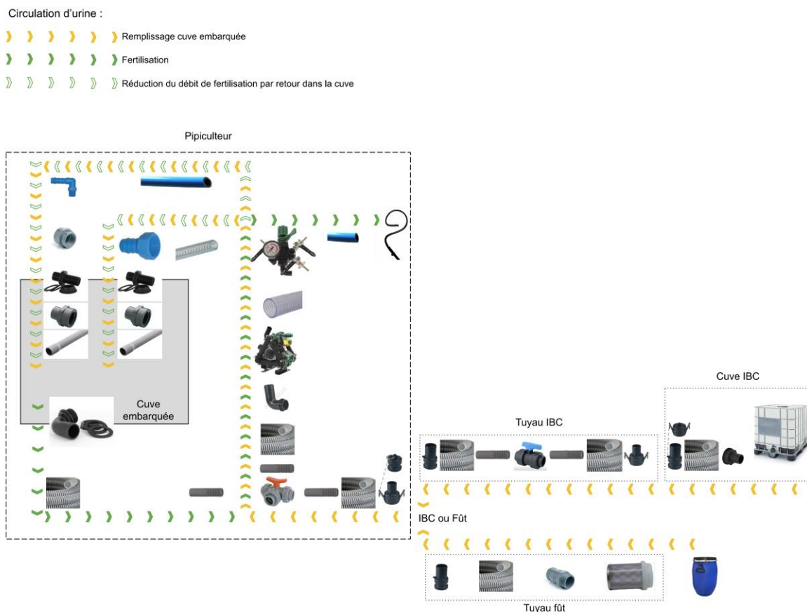
Figure 21 : Schéma de circulation du lisain dans le Pipiculteur. Le remplissage de la cuve embarquée et l'application de lisain dans le sol se font avec la même pompe : c'est l'orientation des vannes qui donne le sens de fonctionnement de la pompe.
