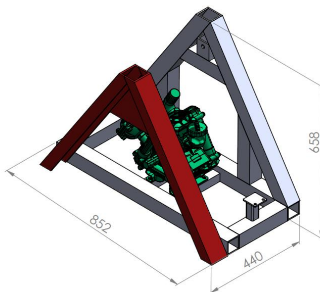
Figure 25 Dimensions de l'adaptateur triangle
