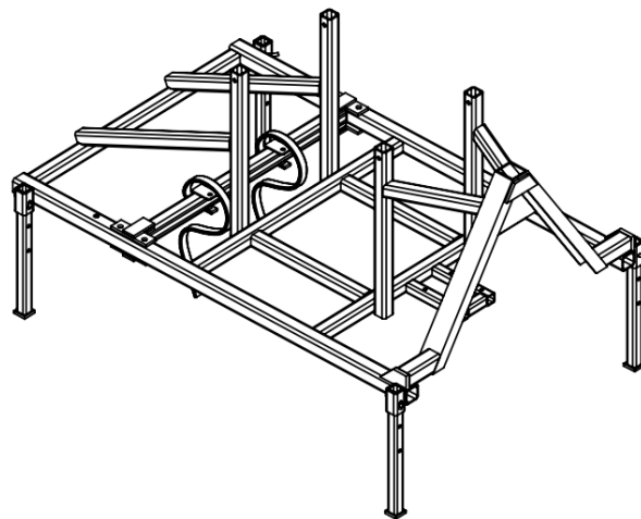
Figure 20 Représentation 3D du châssis du Pipiculteur
