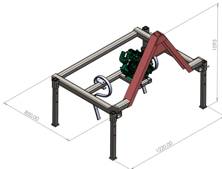
Figure 24 : Dimensions du Pipicuteur sans cuve
