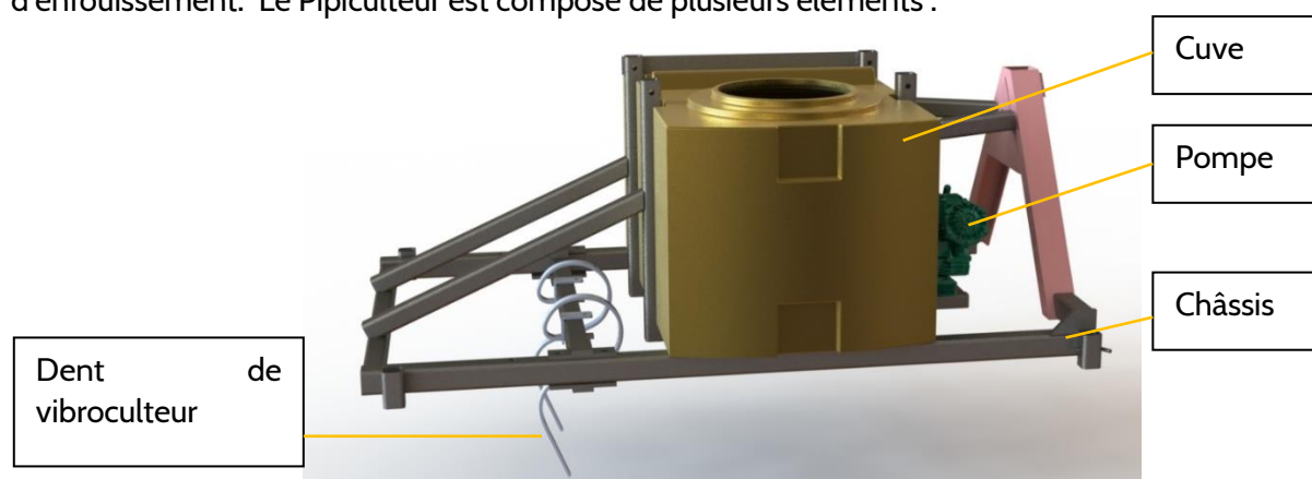
Figure 13 : Modélisation 3D du Pipiculteur
