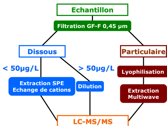
Figure 22 : Protocole en routine de l'analyse du benzalkonium dans les eaux de ruissellement de toiture
