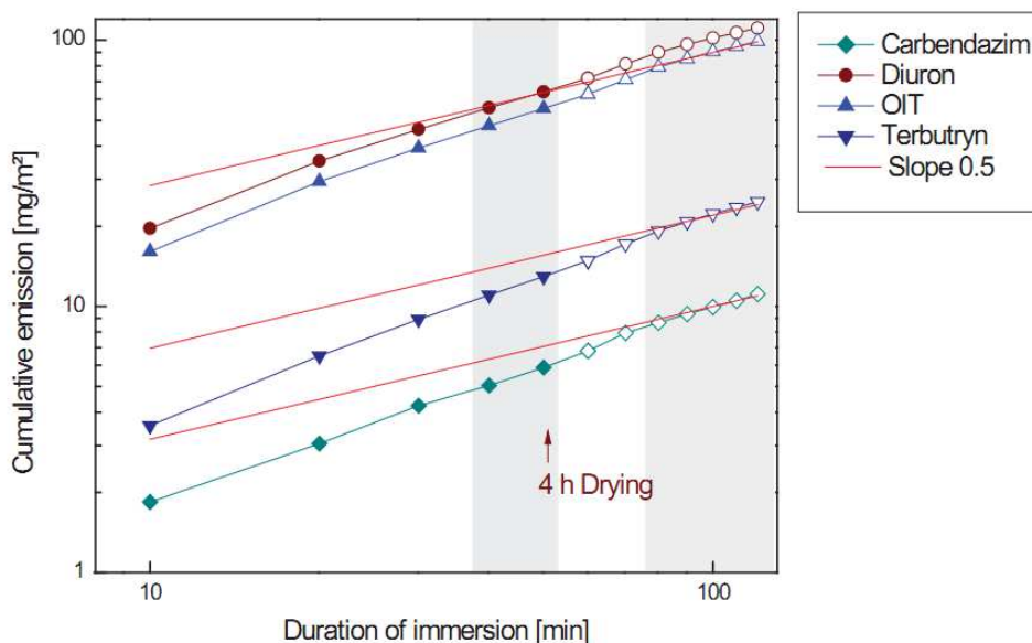
Figure 27 : Emission de biocide cumulée en fonction du temps (échelle "log-log"), une droite de pente 0,5 indique un mécanisme de diffusion (Schoknecht, 2011)
