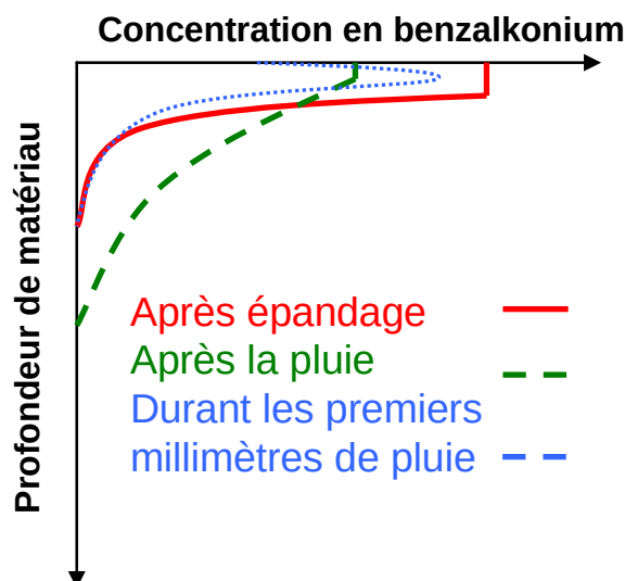
Figure 35 : Evolution possible du gradient de concentration dans le matériau après une pluie
