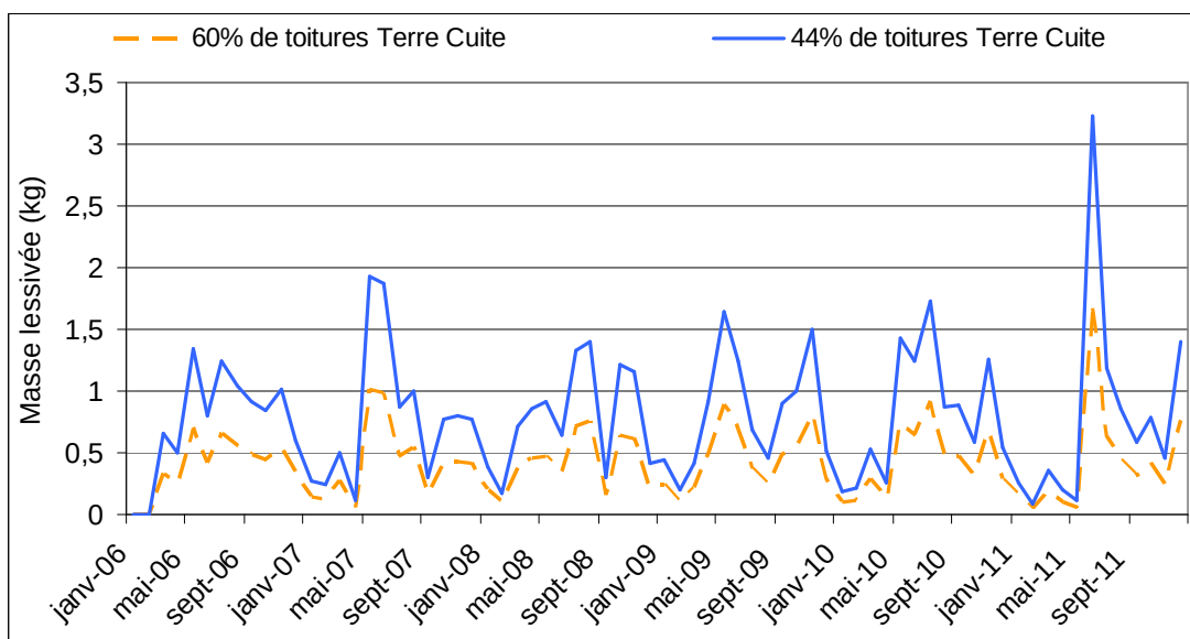
Figure 106 : Evolution de la masse de benzalkonium émise en fonction de la répartition des matériaux de toiture
