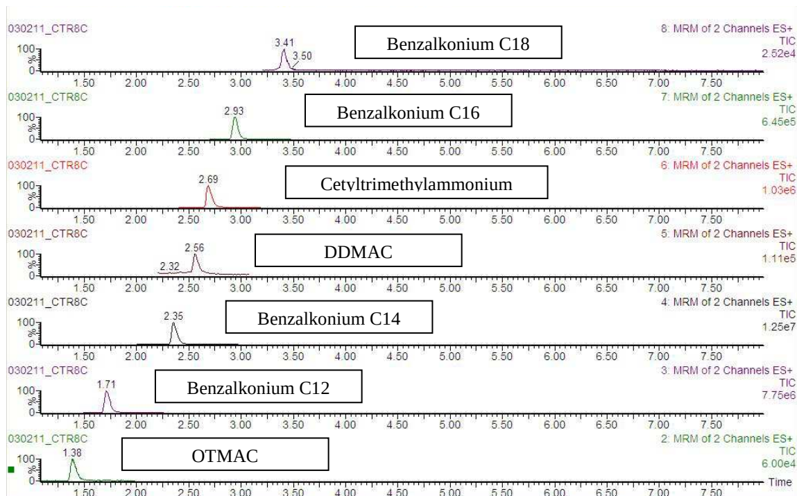
Figure 11 : Chromatogramme obtenu pour un échantillon contrôle
