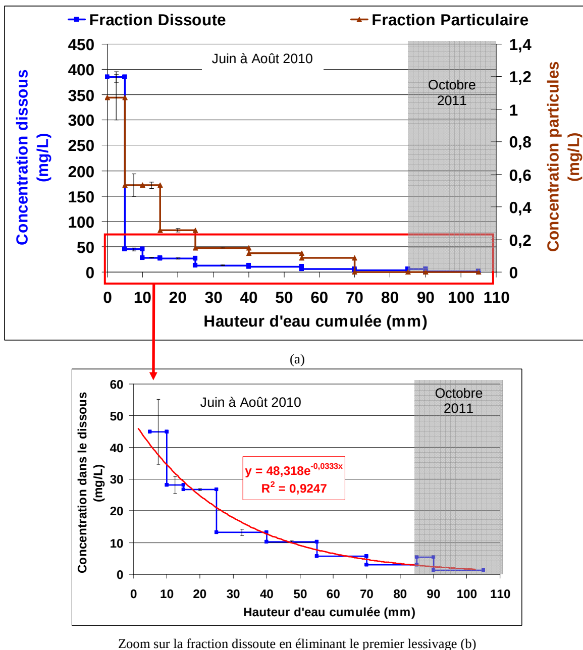
Figure 38 : Concentrations en benzalkonium (C12 + C14) mesurée lors de l'analyse préliminaire
