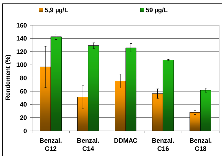
Figure 18 : Rendements d'analyse pour les échantillons non extraits (n = 5, \pm écart type)
