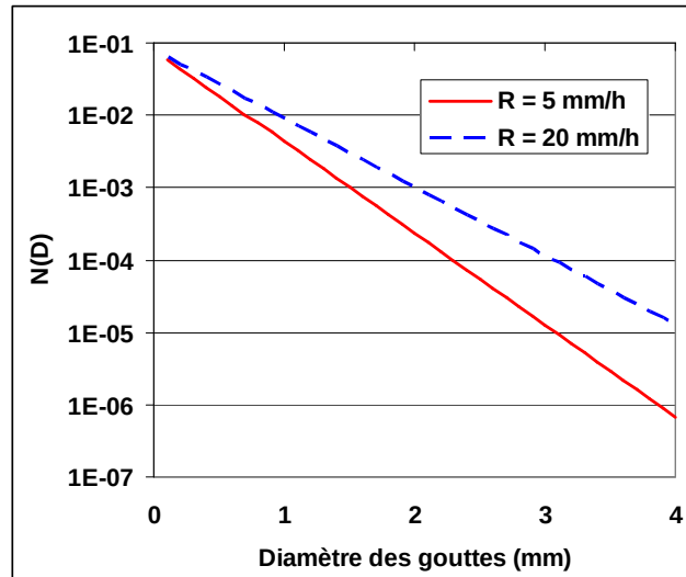
Figure 61 : Distribution granulométrique des gouttes de pluie d'après la relation de (Marshall and Palmer, 1948)
