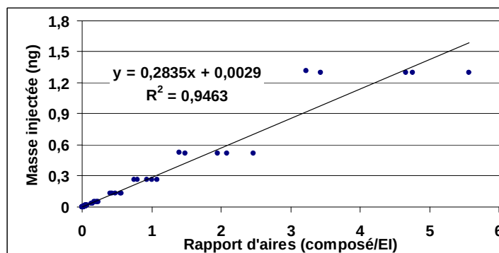
Benzalkonium C14
