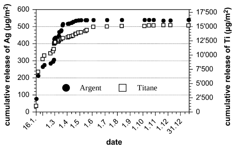
Figure 30 : Evolution de l'émission cumulée d'argent (ronds noirs) et de titane (carrés blancs) issue des façades (Kaegi et al., 2010)
