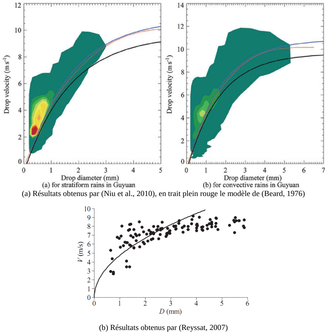
Figure 62 : Relation entre le diamètre des gouttes et la vitesse de chute
