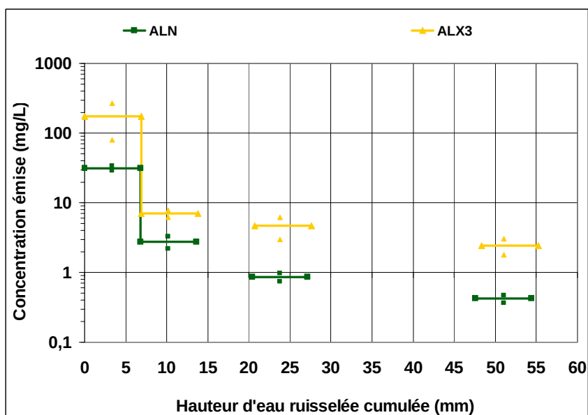
Figure 82 : Evolution de la concentration à l'aval des tuiles terre cuite siliconées à différents dosages
