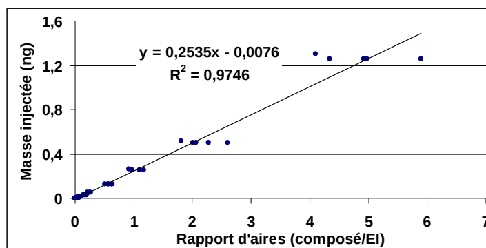
Benzalkonium C18
