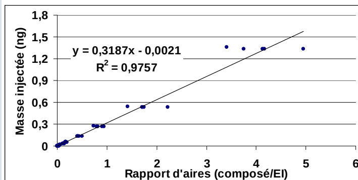
Benzalkonium C12
