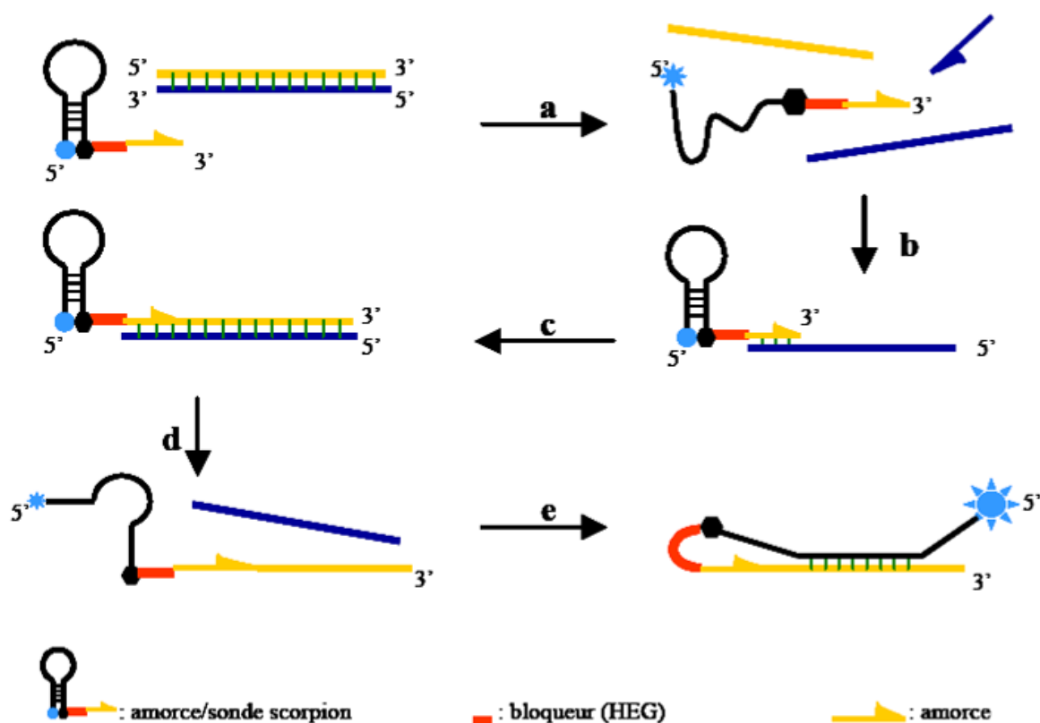
Figure 14 : Déroulement des étapes de dénaturation (a), d'hybridation des amorces PCR (b), d'élargissement (c), de dénaturation secondaire (d) et d'hybridation de la balise moléculaire (e) de la PCR en temps réel par amorce scorpion (Poitras et Houde 2002)
