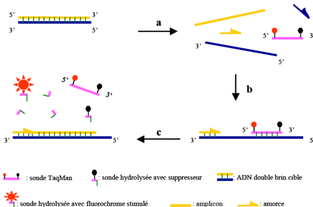
Figure 11 : Conditions et déroulement des étapes de dénaturation (a), d'hybridation des sondes, d'hybridation des amorces PCR (b) et d'elongation (c) de la PCR en temps réel basée sur l'utilisation d'une sonde TaqMan™ (Poitras et Houde 2002)
