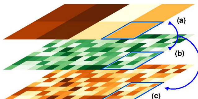
FIGURE 2.3 – Illustration du principe de désagrégation des émissions EMEP : le cadastre à résolution lâche (a) est spatialement désagrégué en exploitant une clef de répartition (b) à une résolution plus fine pour obtenir un cadastre à cette dernière résolution (c).
