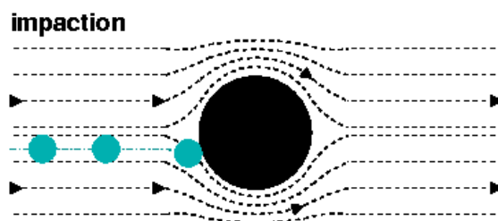
FIGURE 3.2 – Illustration schématisque du processus de collecte par impaction. La particule est transportée par l'écoulement quasi-laminaire puis sort de sa ligne de courant du fait de son inertie et impacte une rugosité de la surface.
