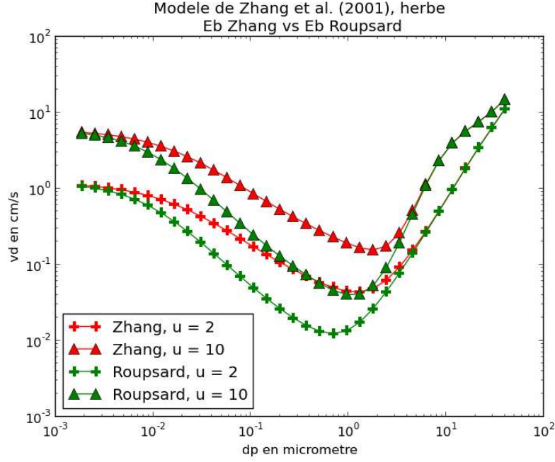
FIGURE 3.6 – Vitesses de dépôts secs en utilisant la valeur du coefficient \gamma proposée dans Zhang et al. (2001) et celle déterminée à partir des expérimentations de Rounsard et al. (2013).
