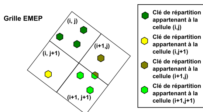
FIGURE 2.2 – Illustration pour une clef de répartition surfacique de l’affectation des éléments de surface aux cellules du cadastre.
