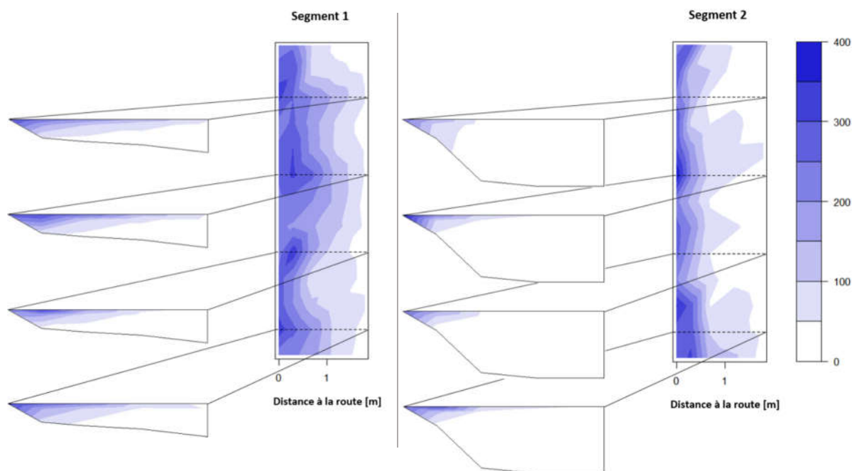
Figure 32 : Cartographie des concentrations en cuivre [mg/kg] à la surface en en profondeur, mesurées sur chacun des deux segments. La route se situe dans la zone x < 0 .
