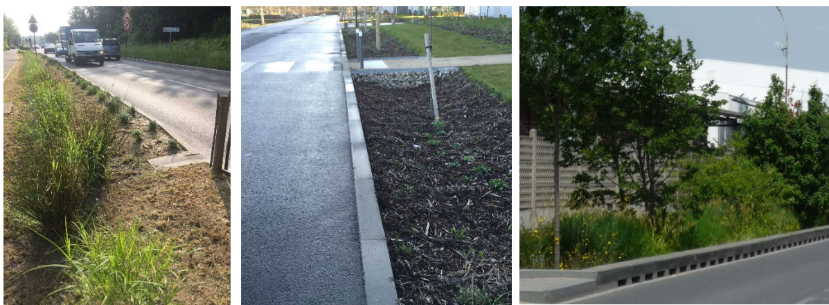
Figure 102 : Exemples d'alimentation en eau de noues en proximité immédiate de la route, aménagements respectivement situés à Torcy, à Montévrain et à Vitry (Gromaire, 2018a)
