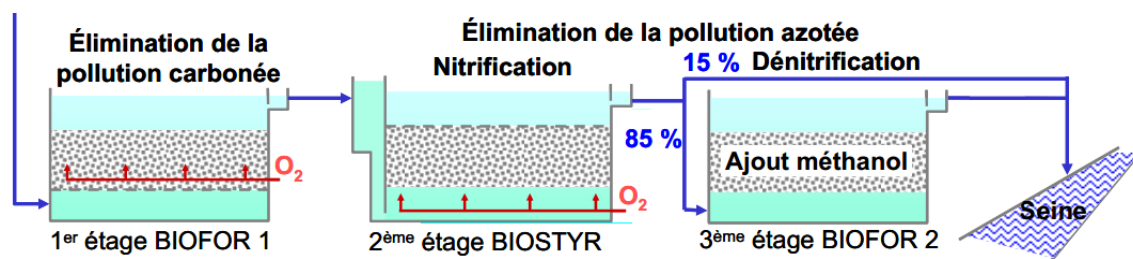
Figure 43 : Traitement par biofiltration dans la station d'épuration de Seine Centre (source Rocher et al., 2006)
