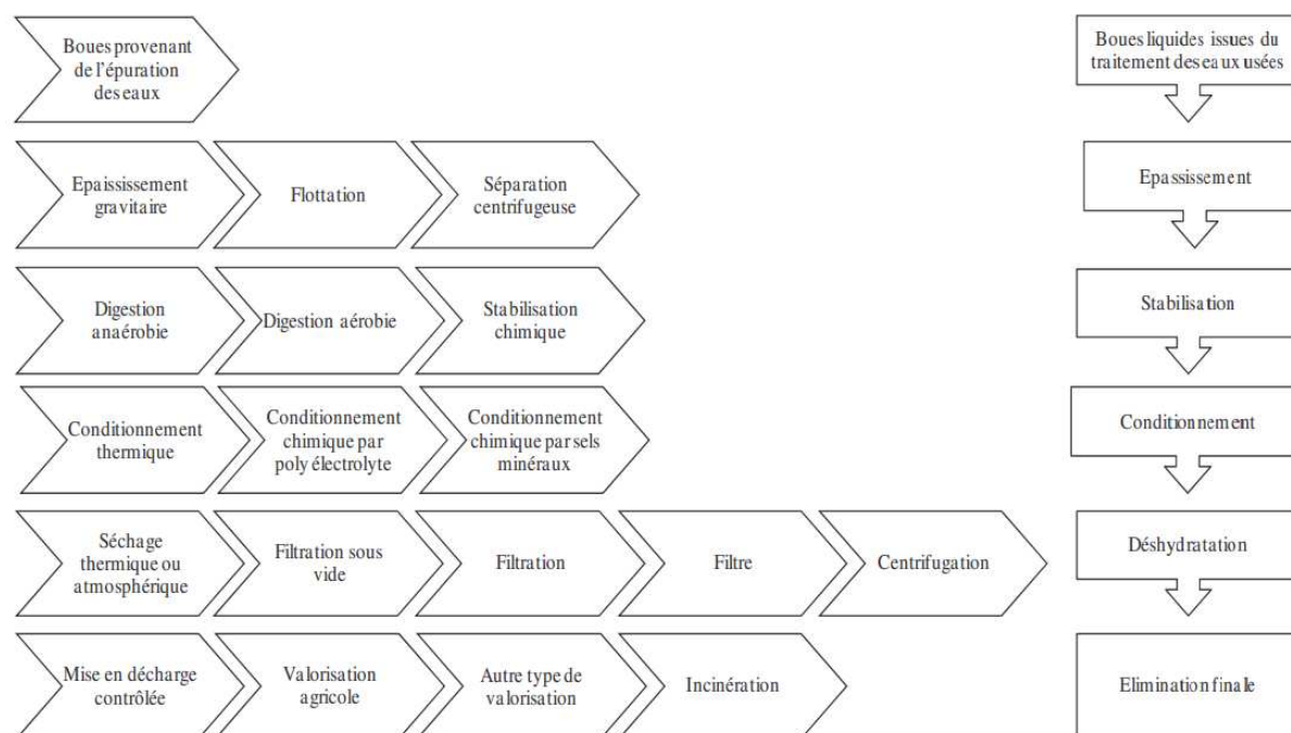
Figure 44 : Traitement des boues de station d'épuration (Perez-Fabiel, 2009)
