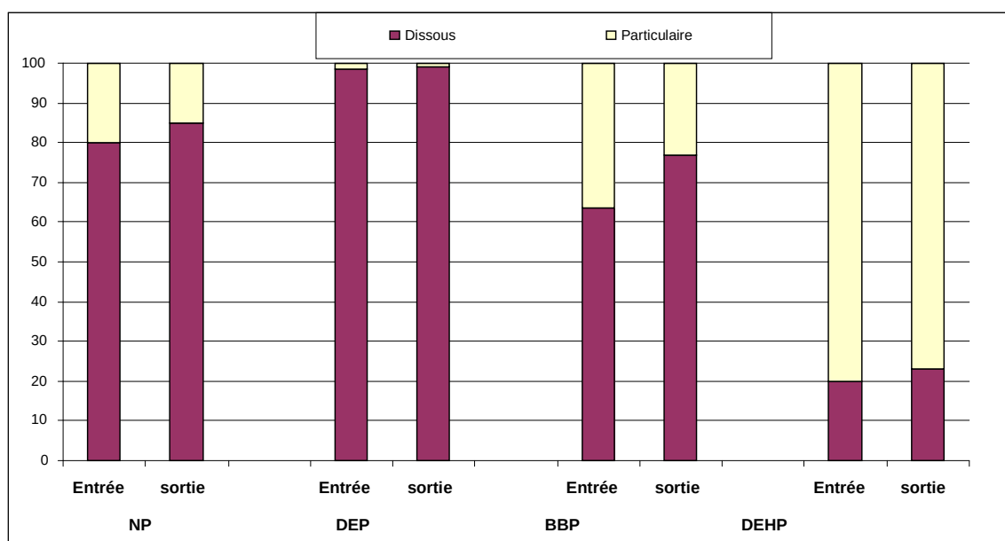
Figure 59 : Répartitions des AP et des PAE entre phases dissoute (D) et particulaire (P) en entrée et sortie de traitement primaire
