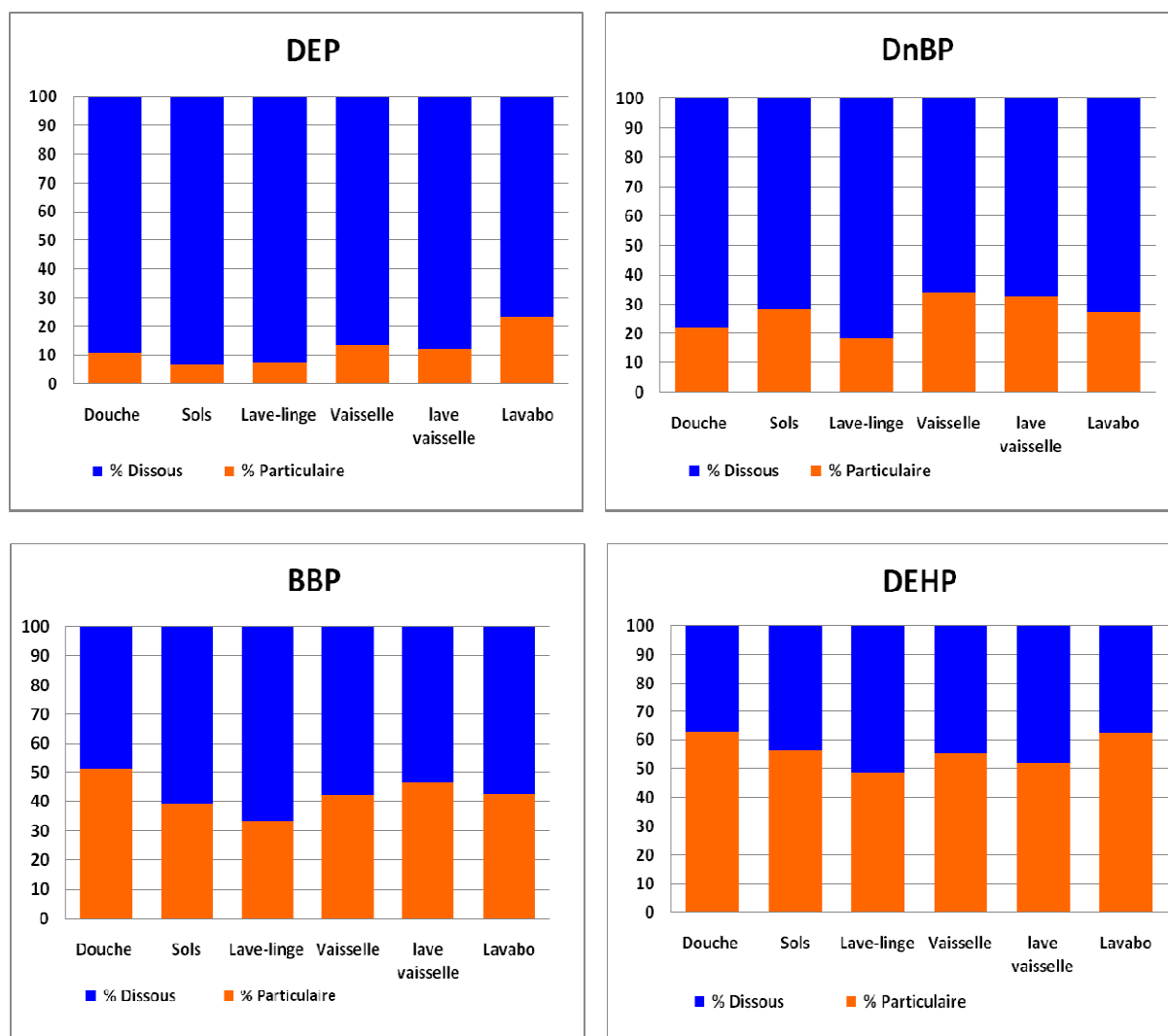
Figure 15 : Répartition des phtalates entre les phases dissoute et particulaire (en %)
