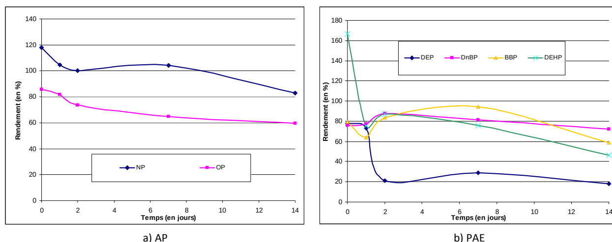
Figure 53 : Evolution des rendements d'extraction a) des AP et b) des PAE en fonction du temps (en %)
