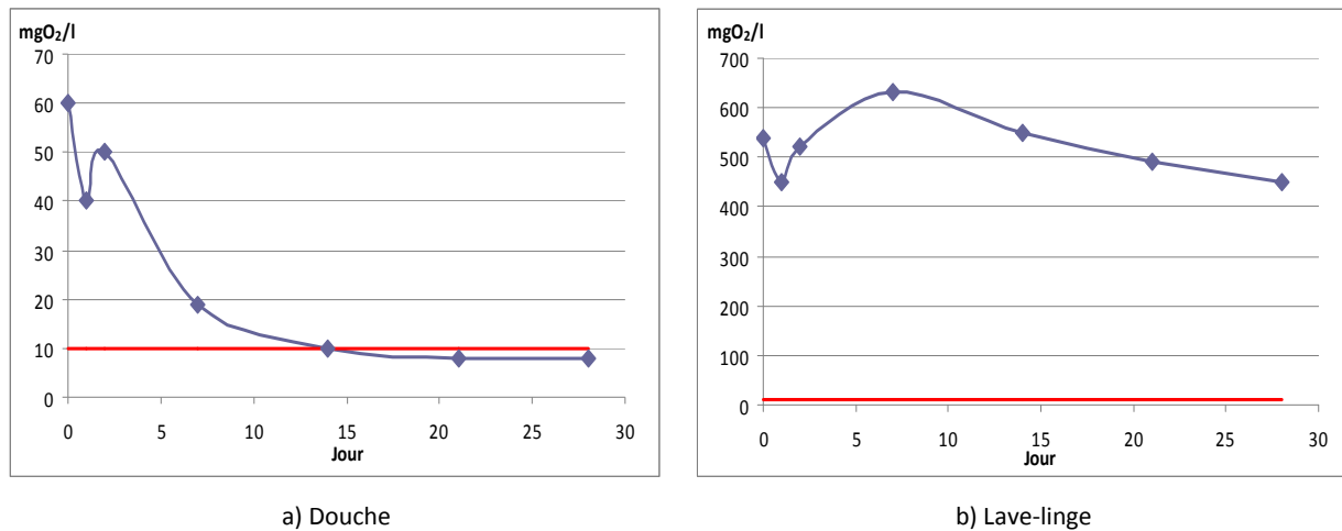
Figure 31 : Evolution de la DBO5 dans les eaux a) de douche et b) de lave-linge au cours du temps
