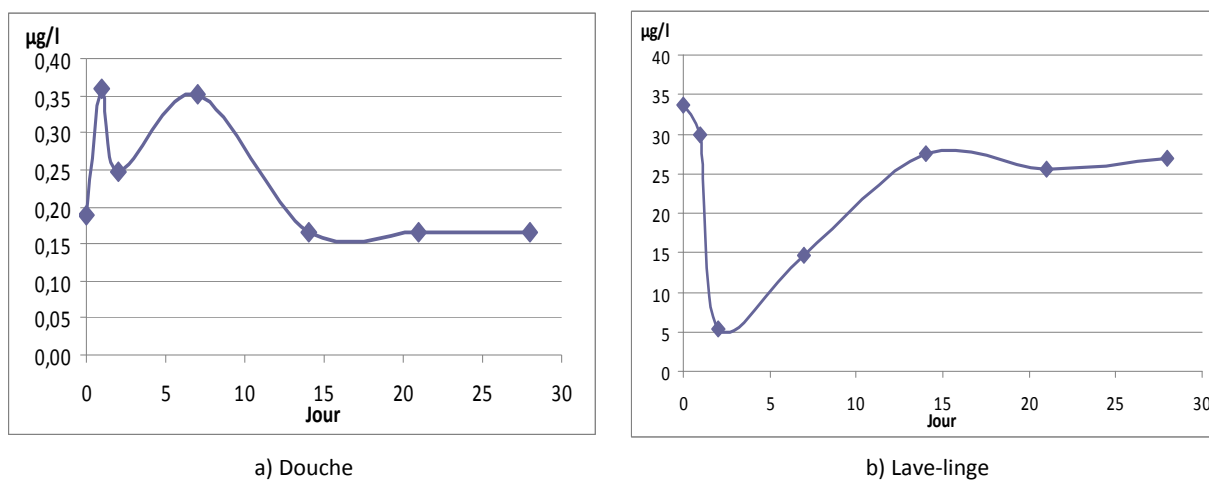
Figure 37 : Evolution des concentrations du BBP dans les eaux a) de douche et b) de lave-linge au cours du temps
