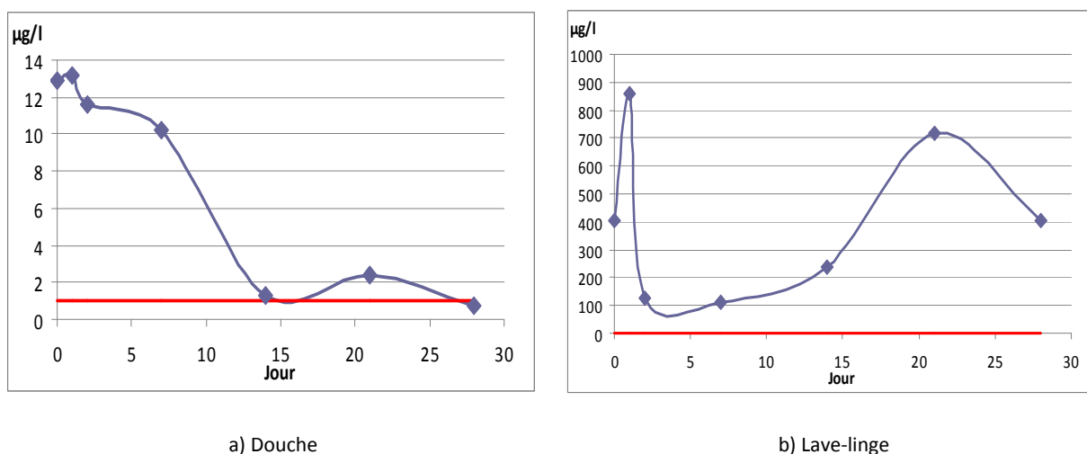
Figure 38 : Evolution des concentrations du DEHP dans les eaux a) de douche et b) de lave-linge au cours du temps
