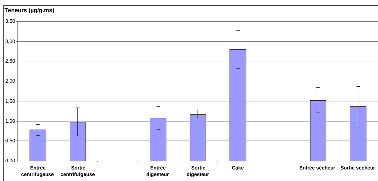
Figure 65 : Teneurs du NP dans les boues de stations d'épuration (µg/g.ms)
